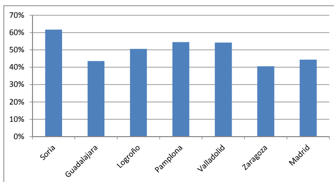
Ahorro energetico electrico sin recup.
