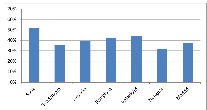
Ahorro energetico electrico con recup.
